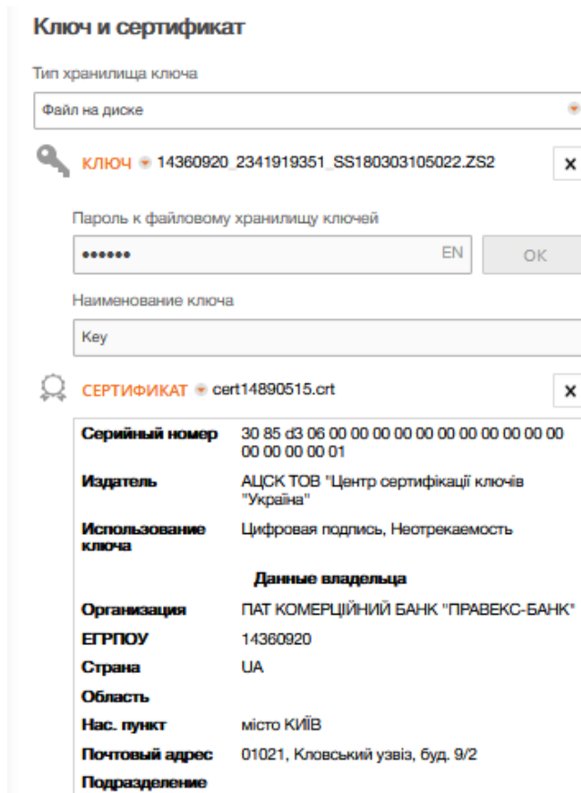
Рис. 9. Ключ і сертифікат після обрання файлів сховища ключа і сертифіката
